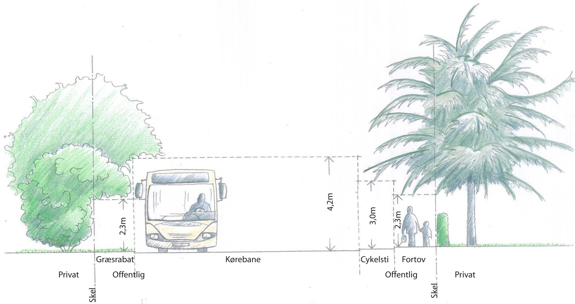
KLIPNING AF HÆKKE, BUSKE OG TRÆER UD TIL OFFENTLIGE AREALER - PRINCIPSNIT
